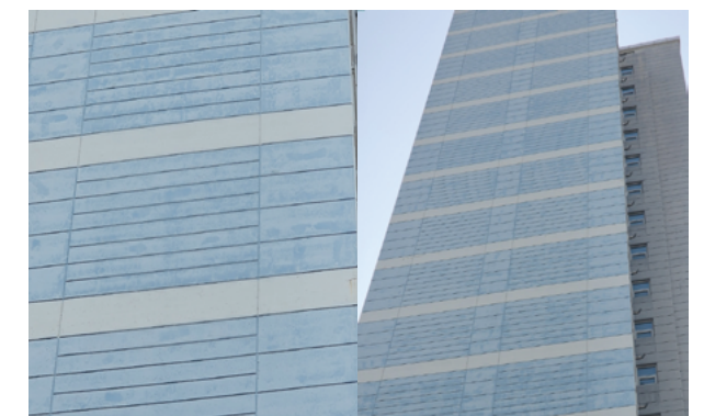
〈 재도장한 지 만 3년 이내에 심각하게 발생한 탈색된 외벽 수성페인트 〉
