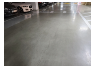
〈 지하주차장 통로 부위 에폭시 라이닝의 아민브러싱 발생으로 탈색되어 있다 〉
